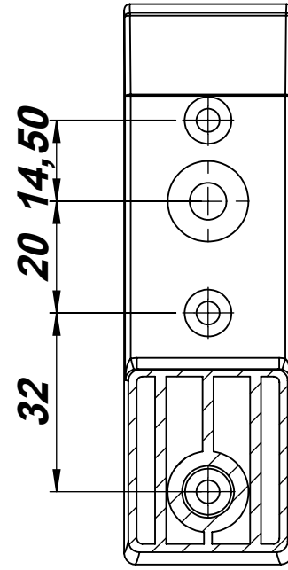
KESİT F-F ÖLÇEK 1 : 1.2
