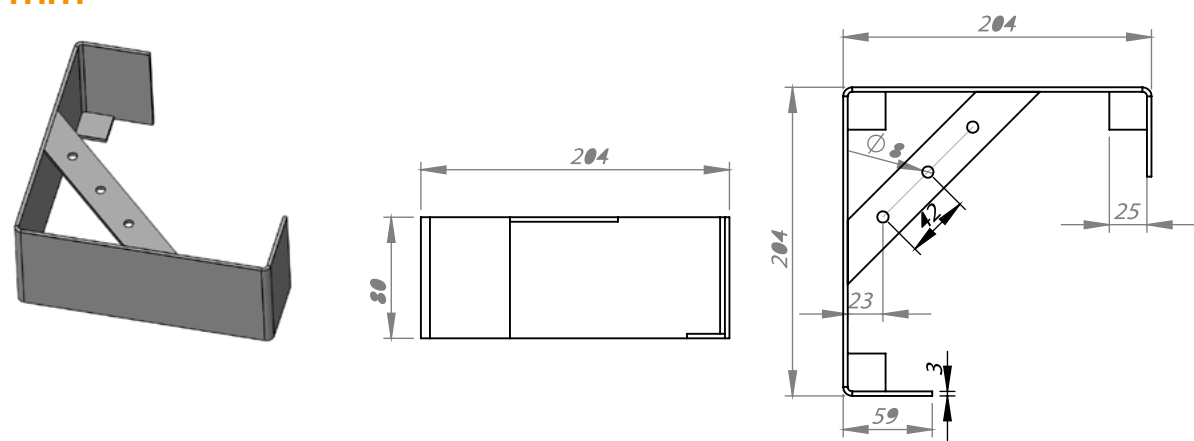
ERH.CNC.03.03 3 mm
