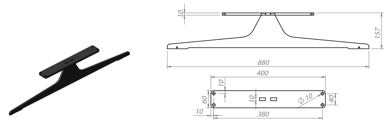
ERH.CNC.10.005 10 mm
