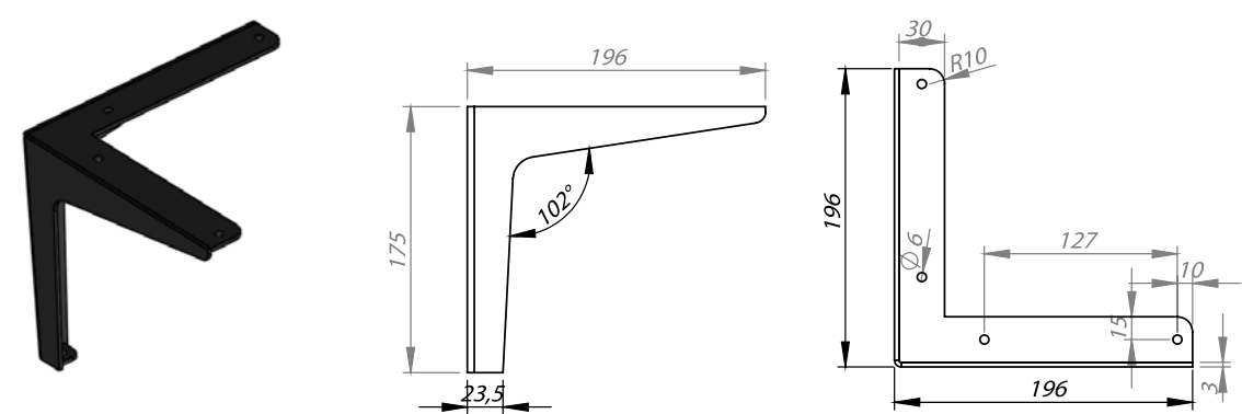
ERH.CNC.03.01 3 mm
