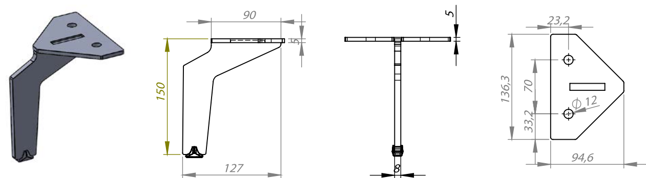
ERH.CNC.08.11 8 mm
