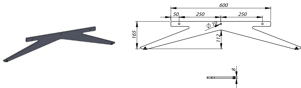
ERH.CNC.08.10 8 mm
