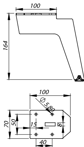
ERH.CNC.08.03 8 mm
