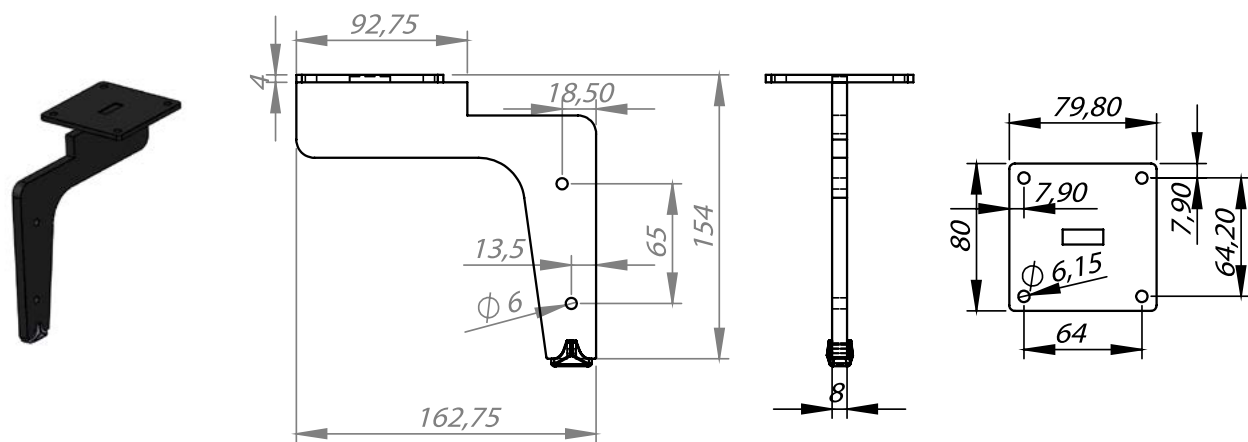
ERH.CNC.08.08 8 mm
